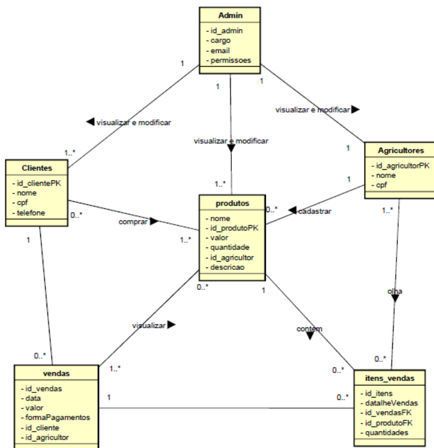
Figura 33 - Modelo Entidade-Relacionamento
